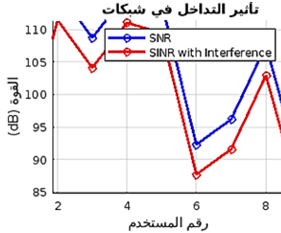
شكل رقم 1. التداخل في شبكات 5ghz
